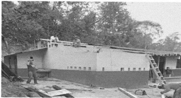
Foto 5: Cocina, sustitucion de vigas de madera por vigas de metal en el area de la cocina.
